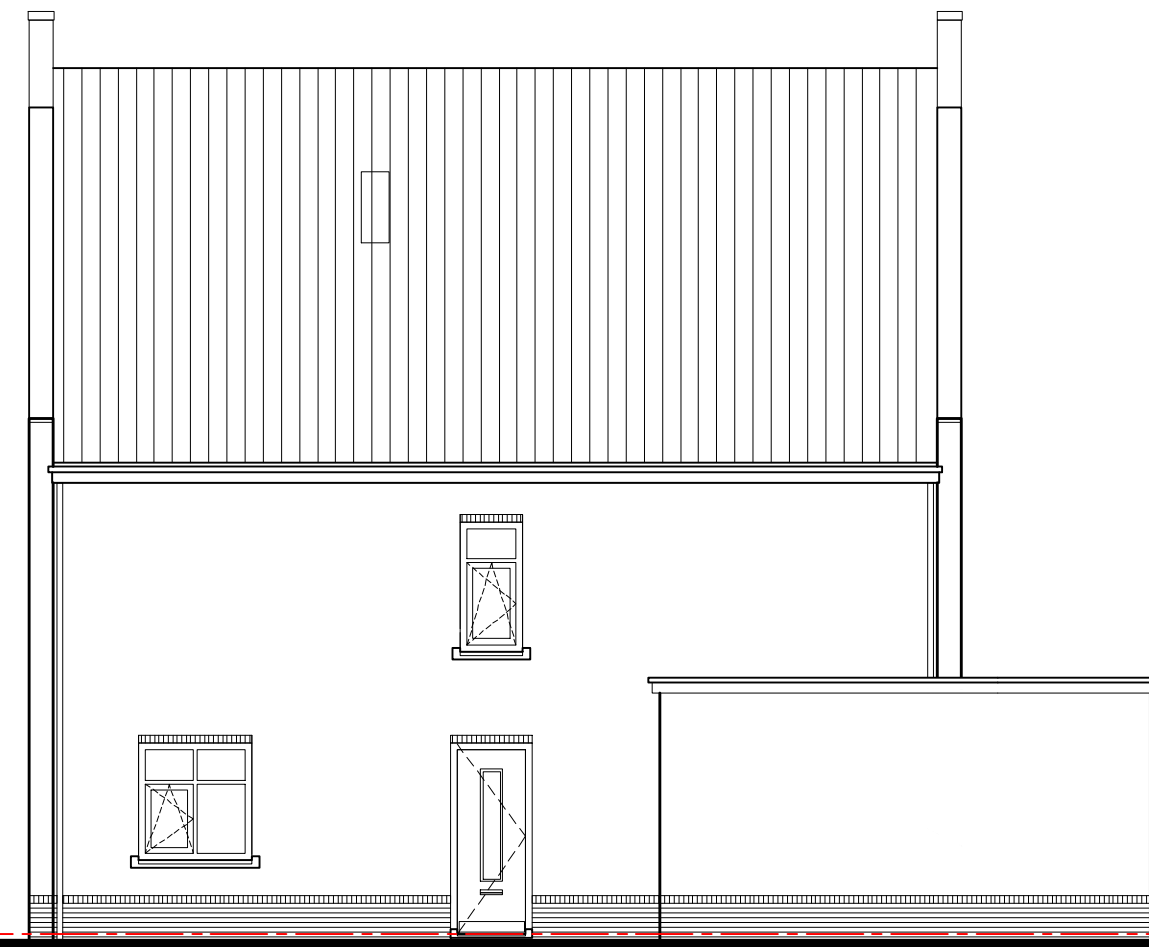
rechter zijgevel
