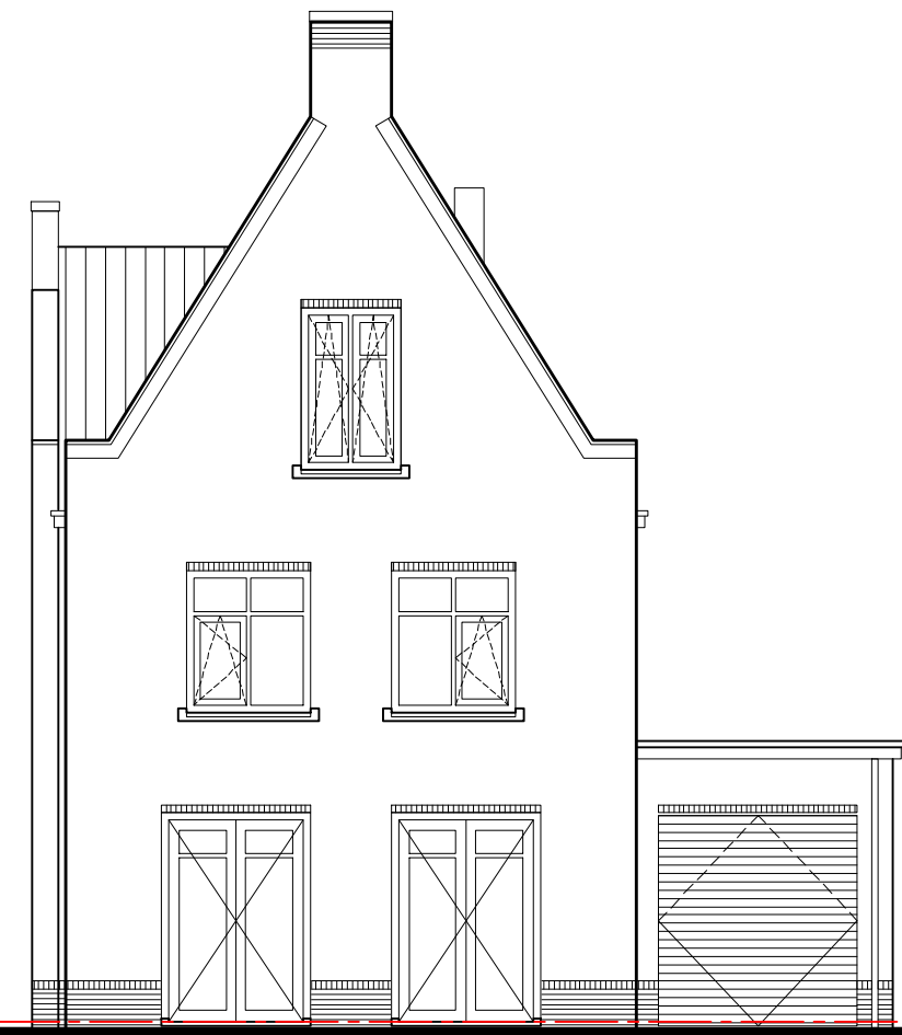
voorgevel
