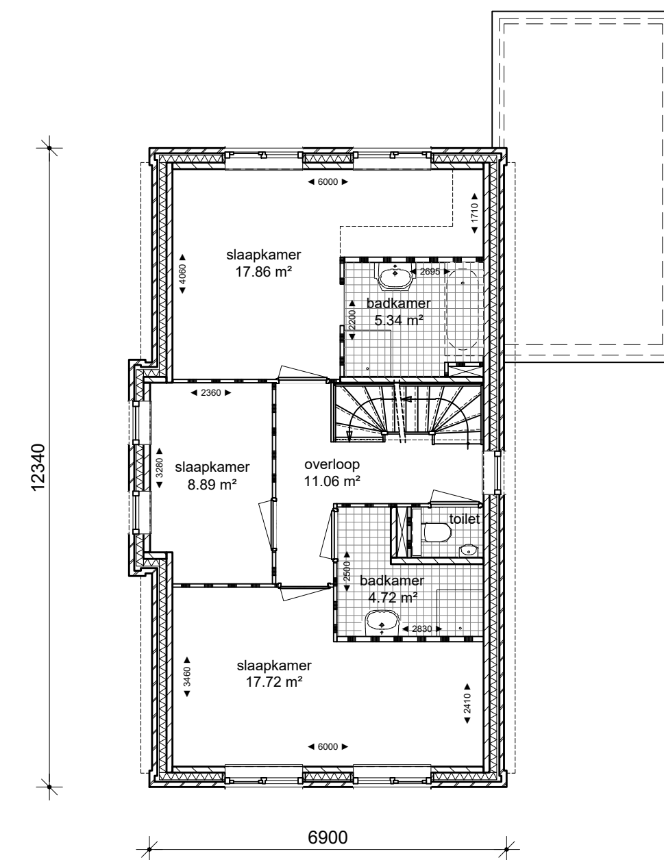
verdieping
