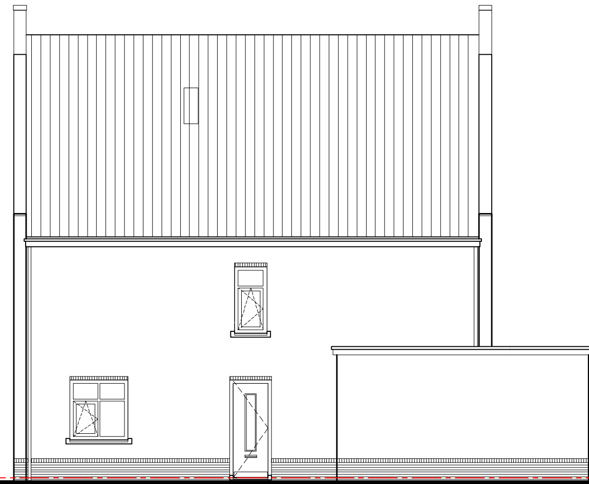
rechter zijgevel
