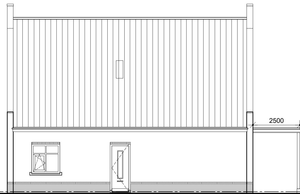
rechter zijgevel
