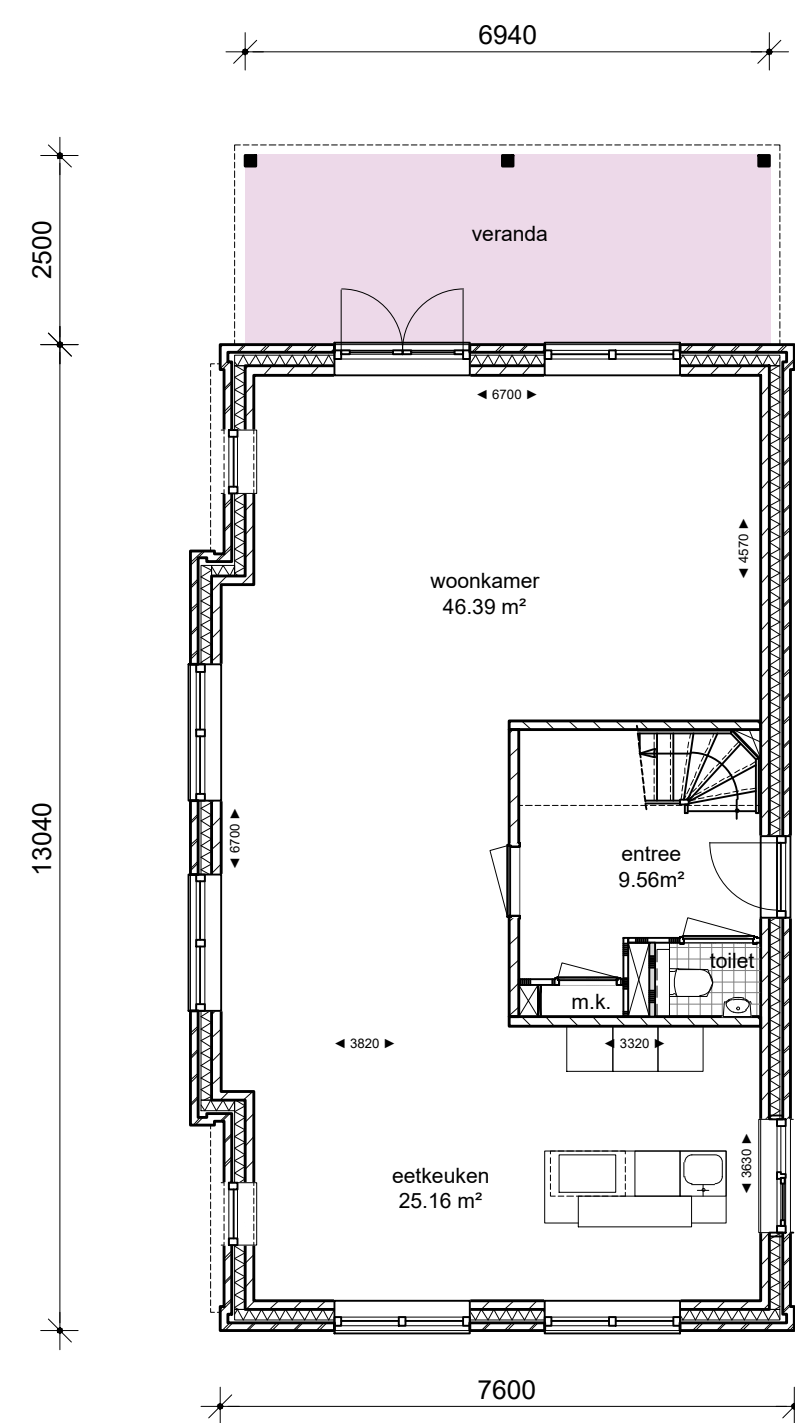
begane grond
