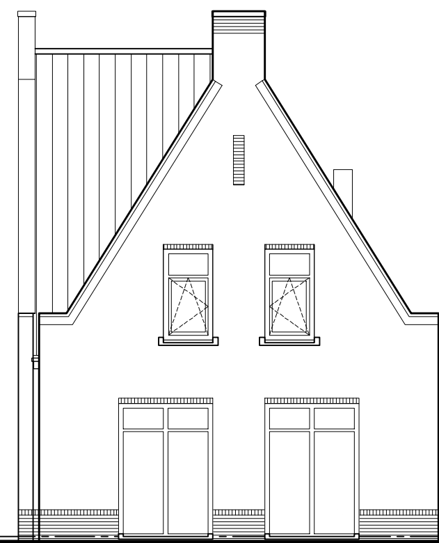
voorgevel
