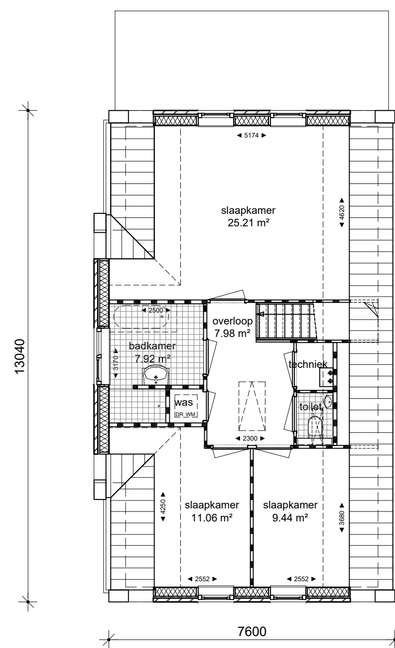
verdieping
