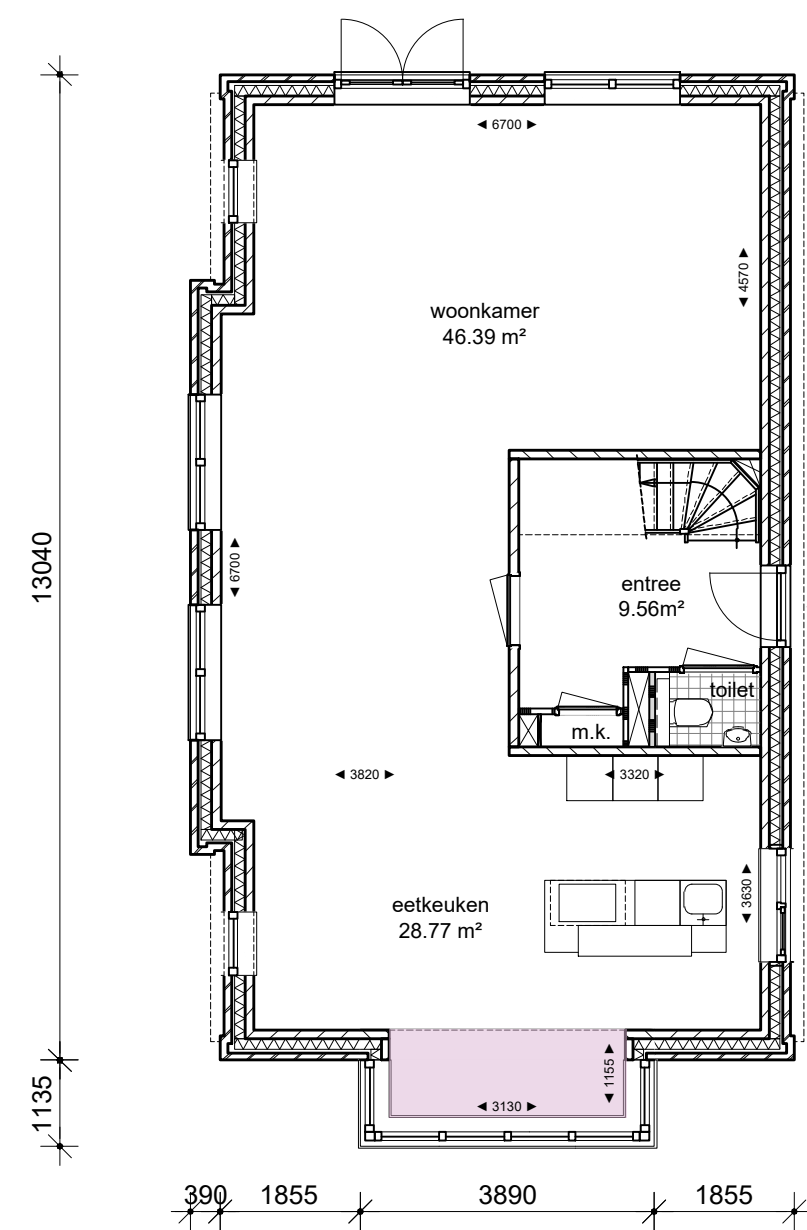
begane grond
