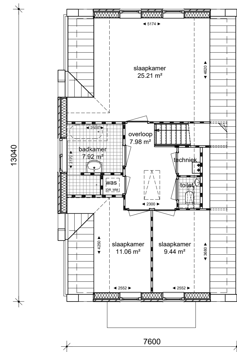
verdieping
