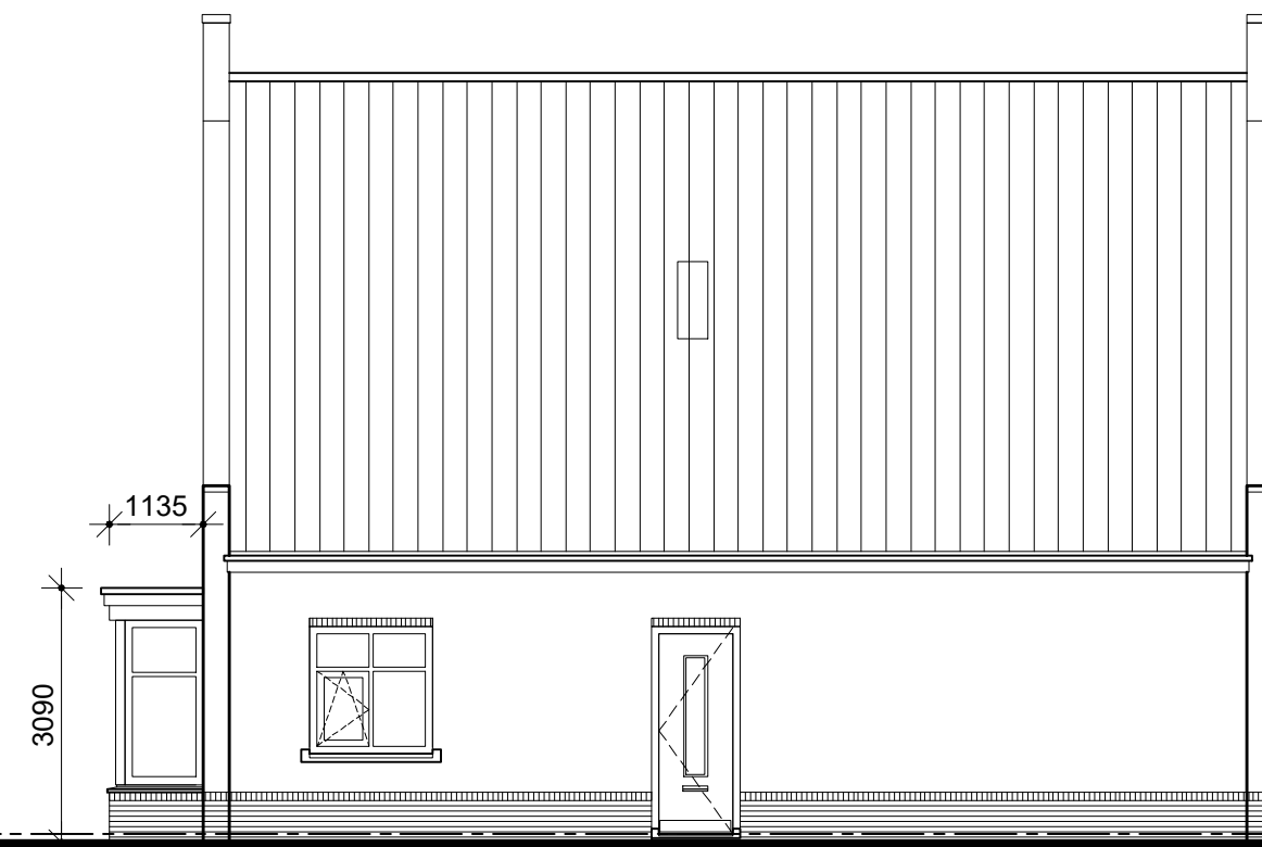
rechter zijgevel
