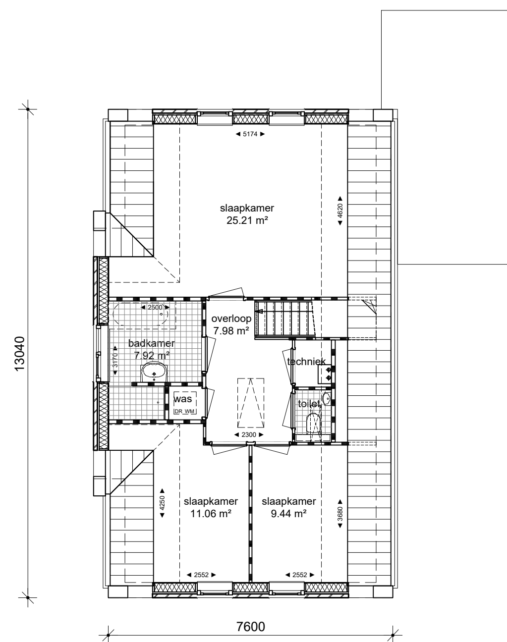
verdieping
