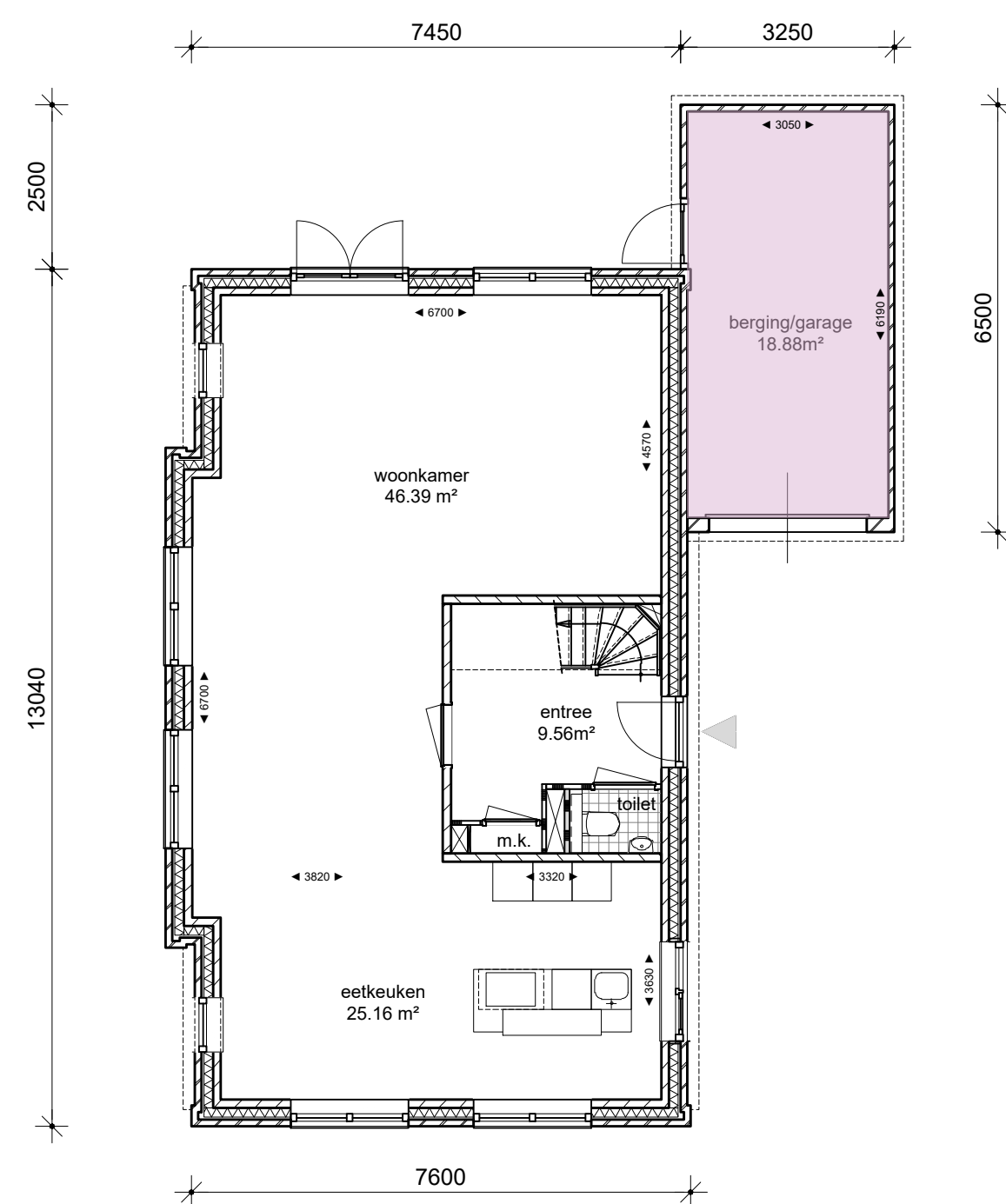
begane grond
