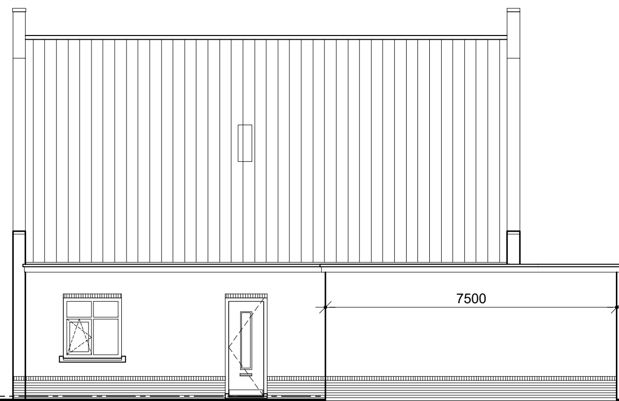
linker zijgevel
