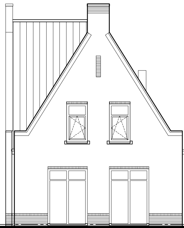
voorgevel
