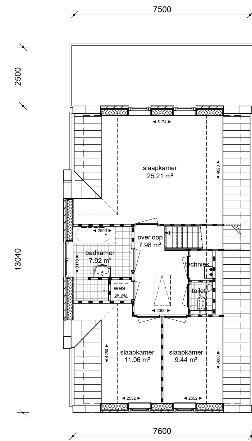
verdieping
