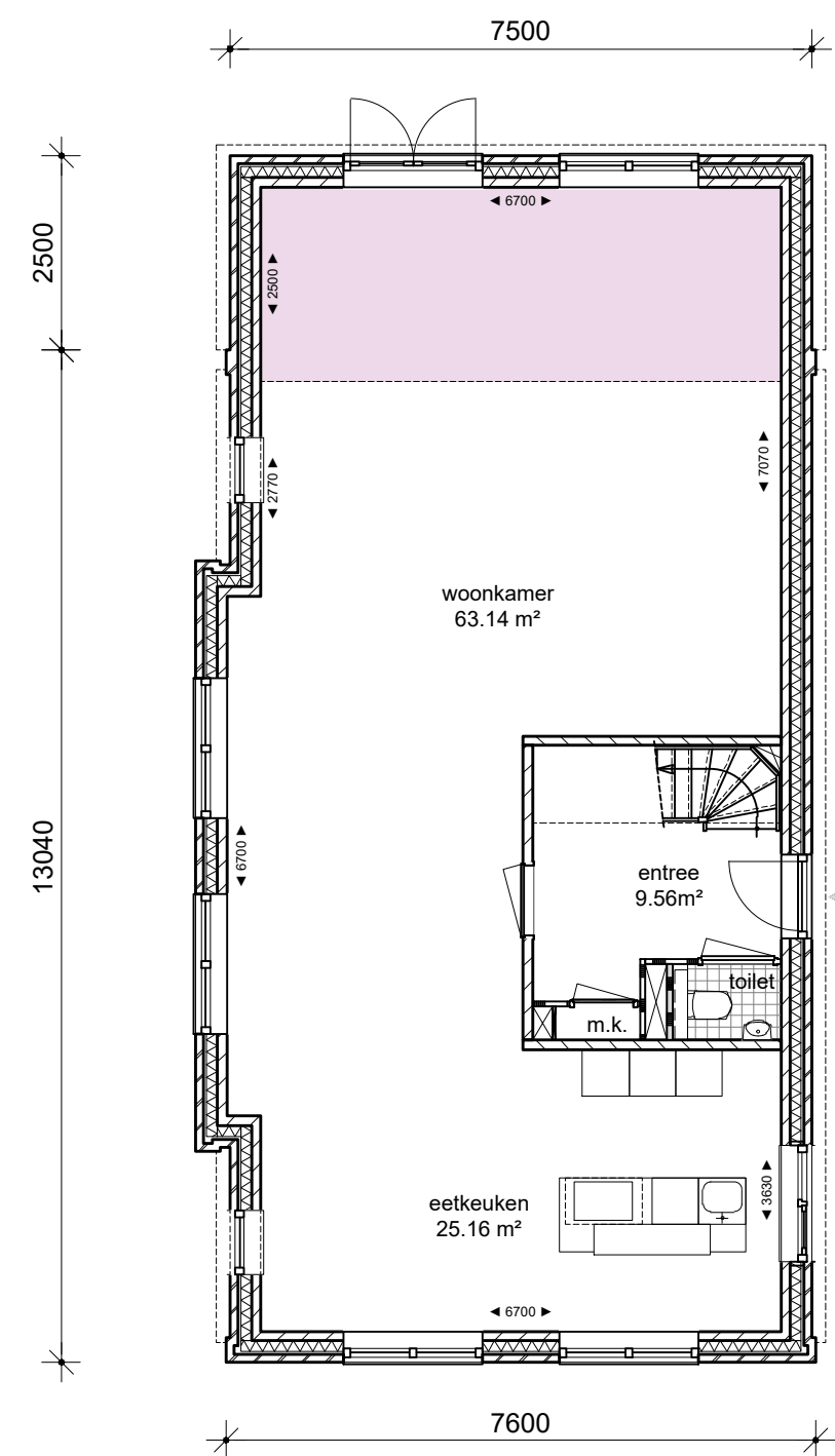
begane grond
